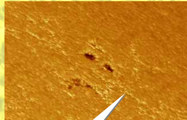
Faculae
