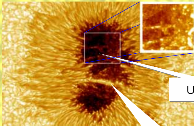
Sonnenfleck
