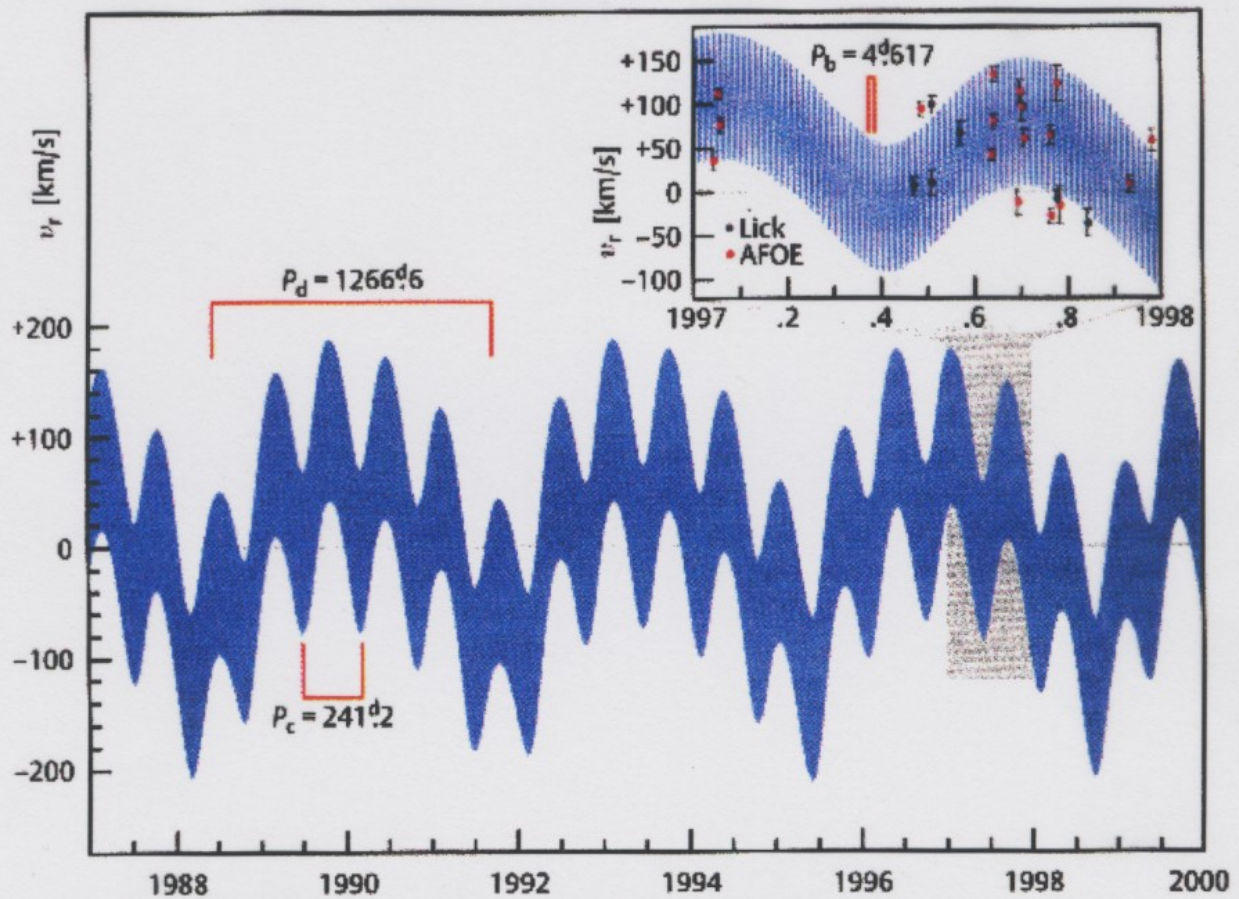
Abb. 9: Die den Messpunkten angepasste Radialgeschwindigkeitskurve von \nu Andromedae lässt sich als Überlagerung von drei Perioden darstellen – 4.6 Tage (vgl. den vergrößerten Ausschnitt), 241 Tage und 3.47 Jahre. (Butler et al. 1999)
